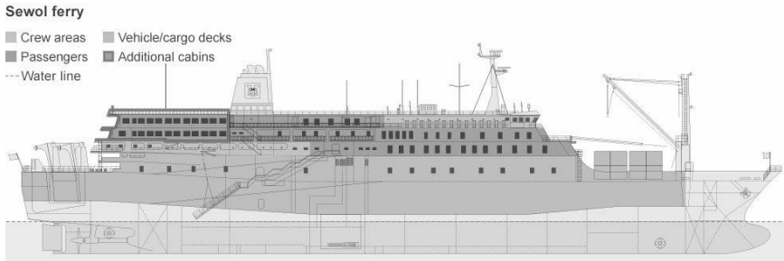
Gráfico 1: Distribución de las áreas en el ferry Sewol
